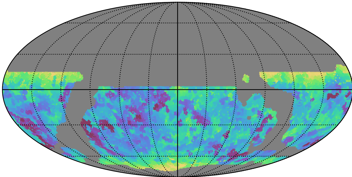
weather_cloudso14v3.4_10yrs WFD i band: Min seeingEff
