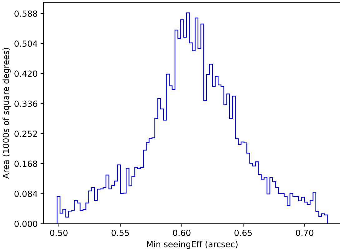
weather_cloudso14v3.4_10yrs WFD i band: Min seeingEff
