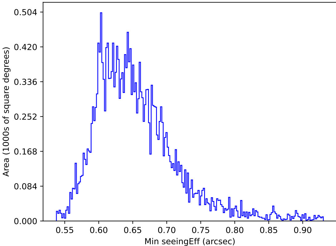
weather_cloudso14v3.4_10yrs All sky y band: Min seeingEff
