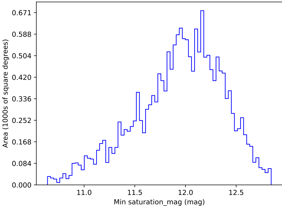
weather_cloudso14v3.4_10yrs WFD z band: Min saturation_mag
