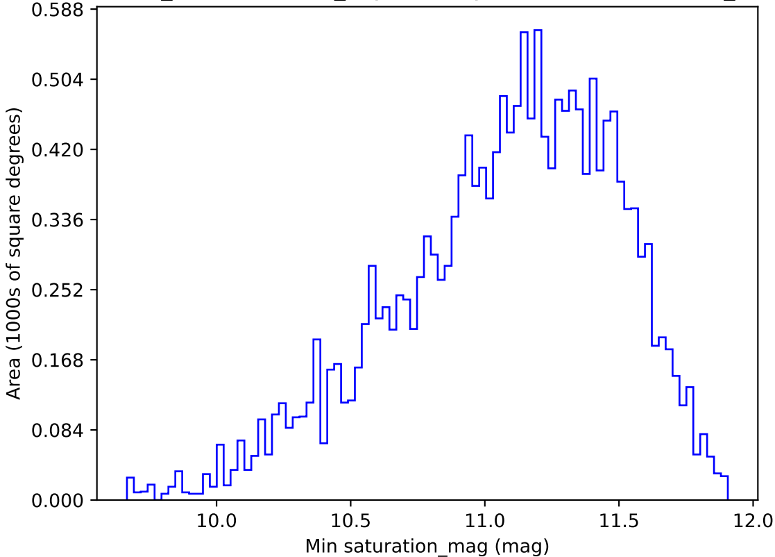
weather_cloudso14v3.4_10yrs WFD y band: Min saturation_mag
