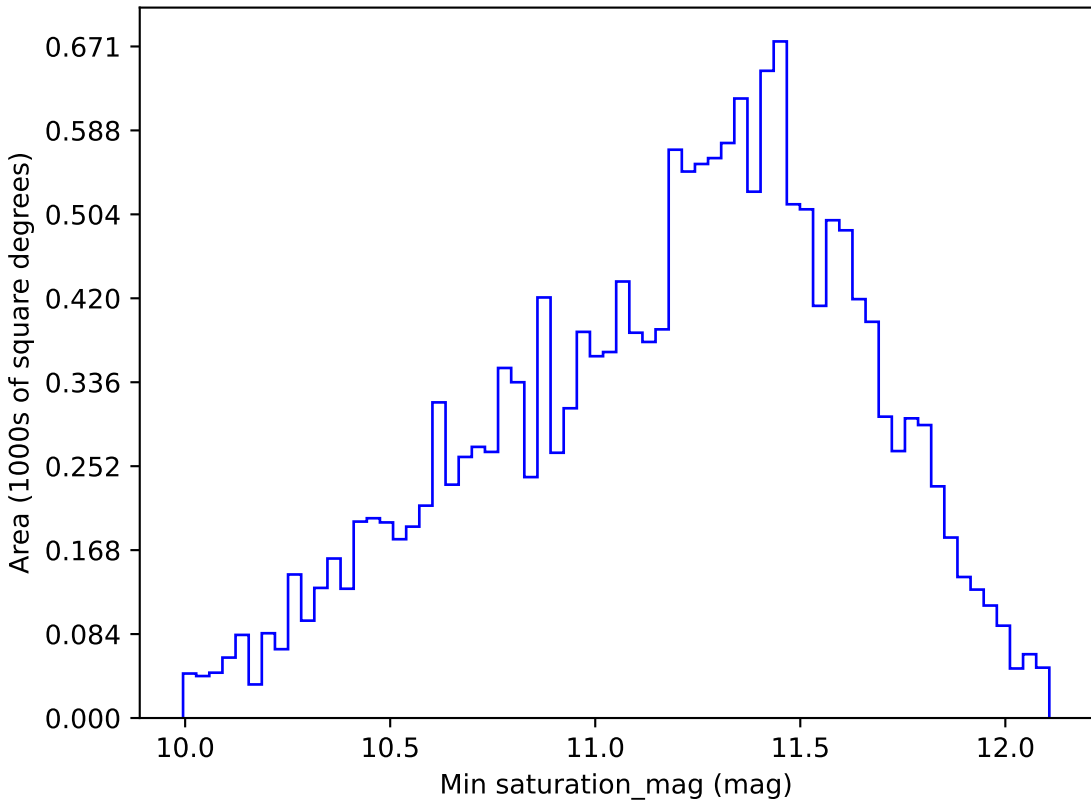
weather_cloudso14v3.4_10yrs WFD u band: Min saturation_mag
