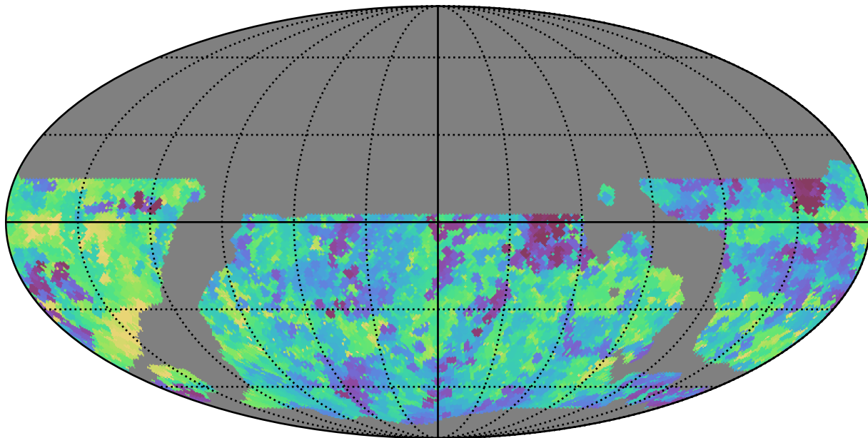
weather_cloudso14v3.4_10yrs WFD r band: Min saturation_mag
