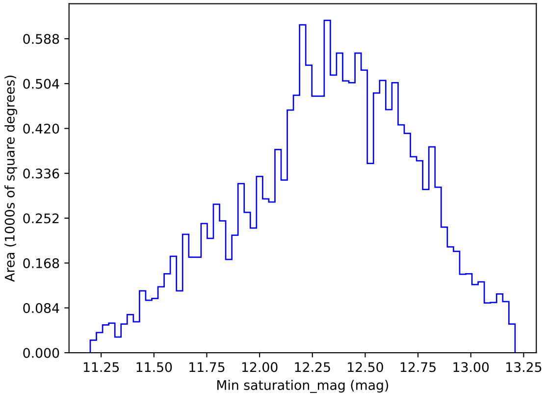
weather_cloudso14v3.4_10yrs WFD r band: Min saturation_mag
