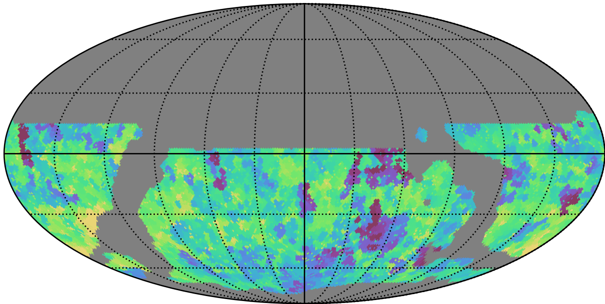
weather_cloudso14v3.4_10yrs WFD i band: Min saturation_mag
