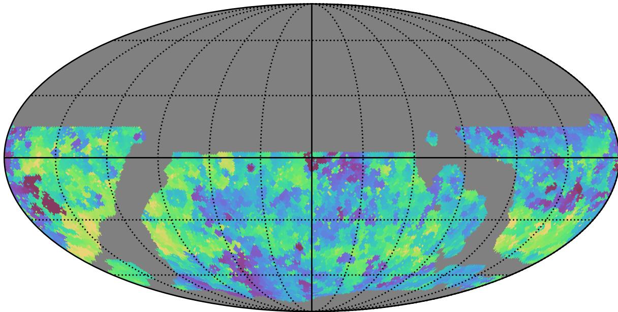
weather_cloudso14v3.4_10yrs WFD g band: Min saturation_mag
