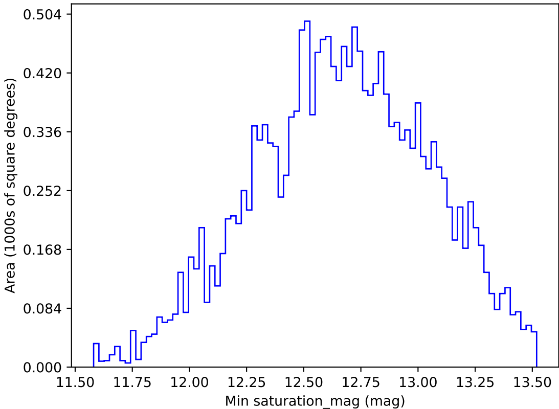
weather_cloudso14v3.4_10yrs WFD g band: Min saturation_mag
