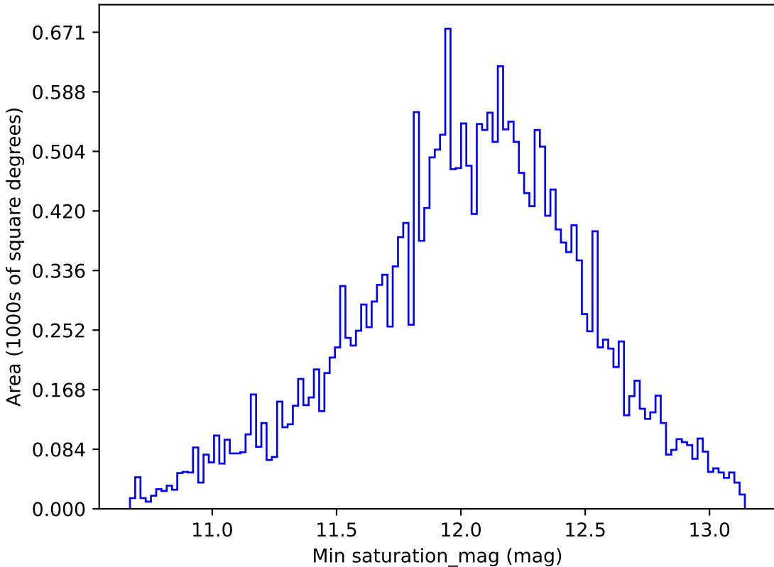
weather_cloudso14v3.4_10yrs All sky z band: Min saturation_mag
