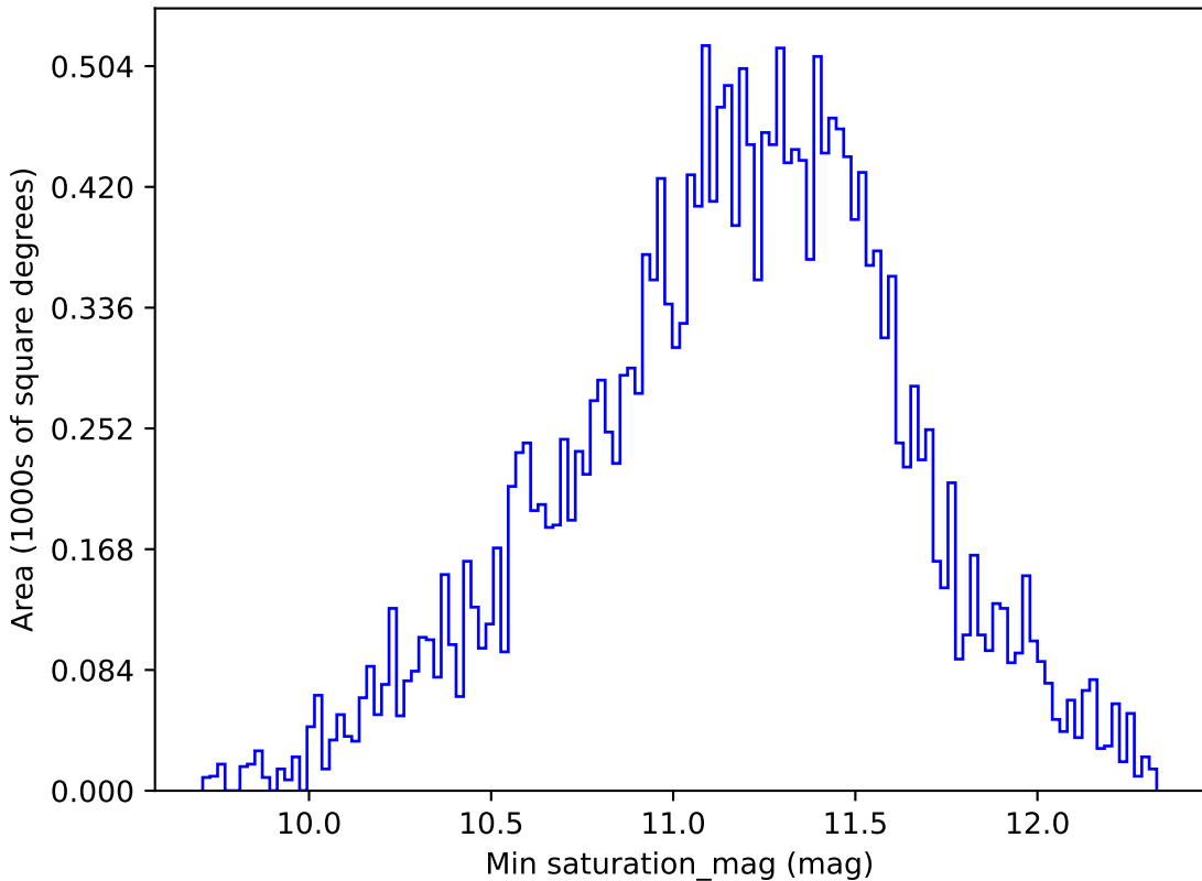
weather_cloudso14v3.4_10yrs All sky y band: Min saturation_mag
