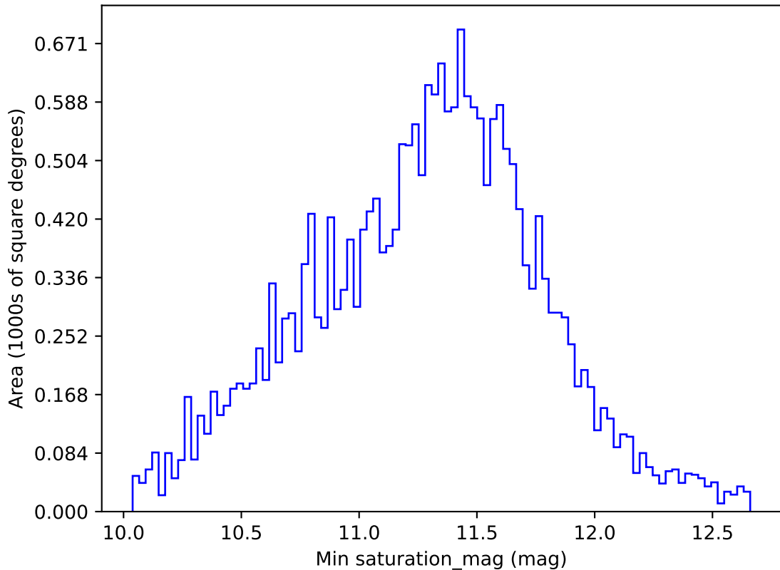
weather_cloudso14v3.4_10yrs All sky u band: Min saturation_mag
