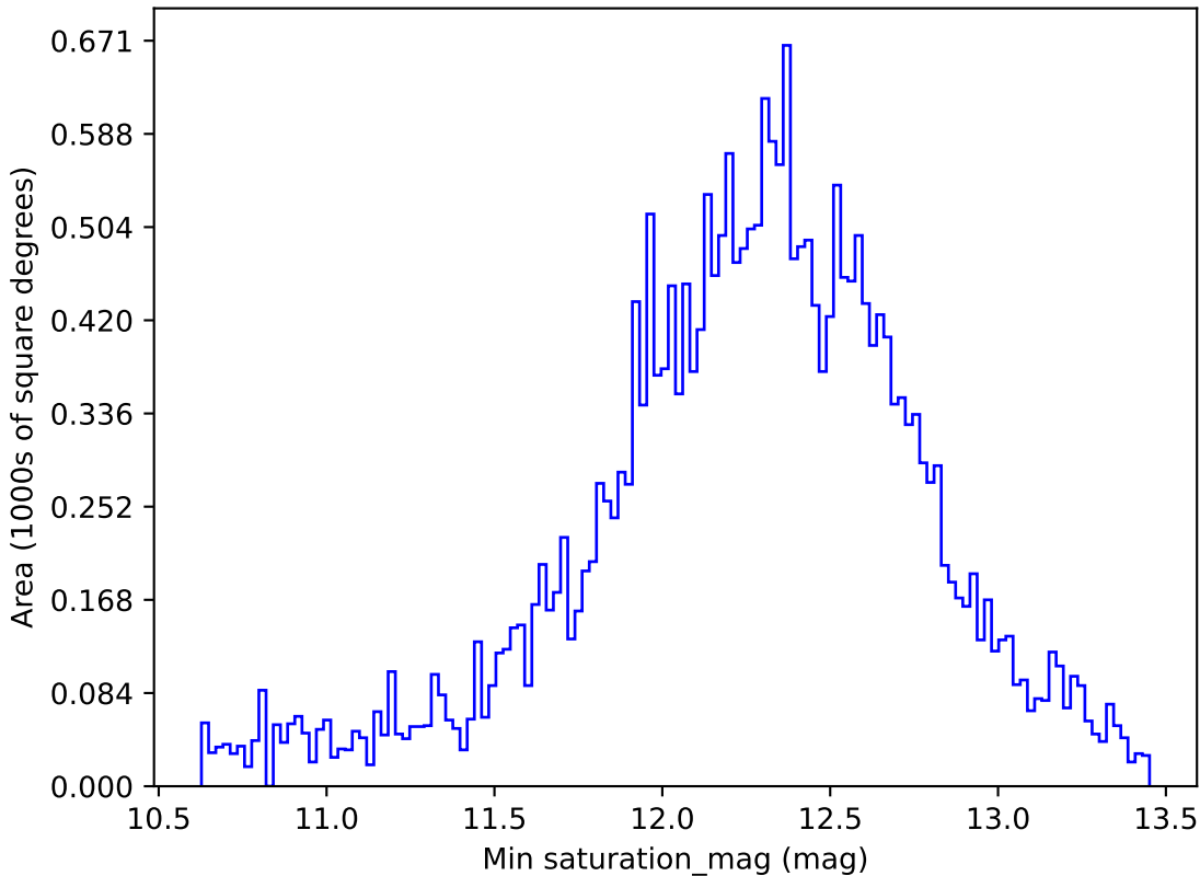
weather_cloudso14v3.4_10yrs All sky i band: Min saturation_mag
