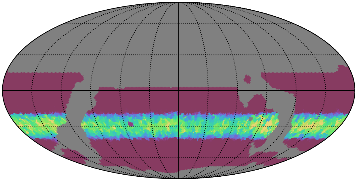
weather_cloudso14v3.4_10yrs WFD y band: Min normairmass
