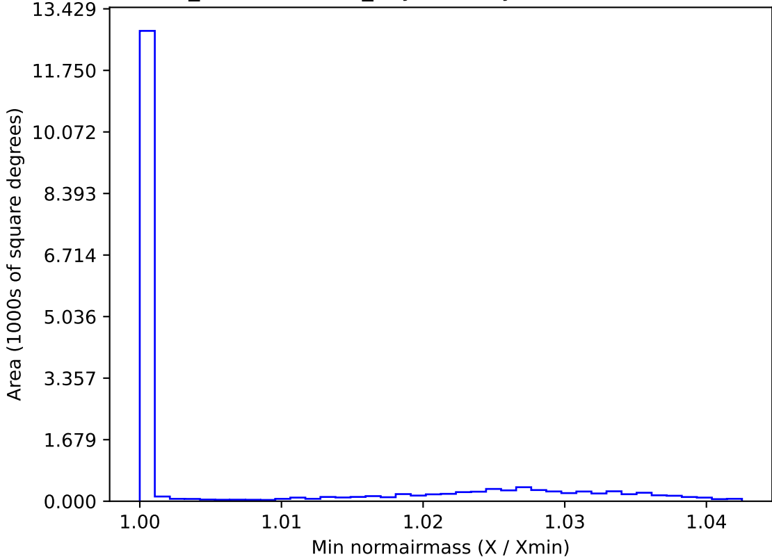
weather_cloudso14v3.4_10yrs WFD y band: Min normairmass
