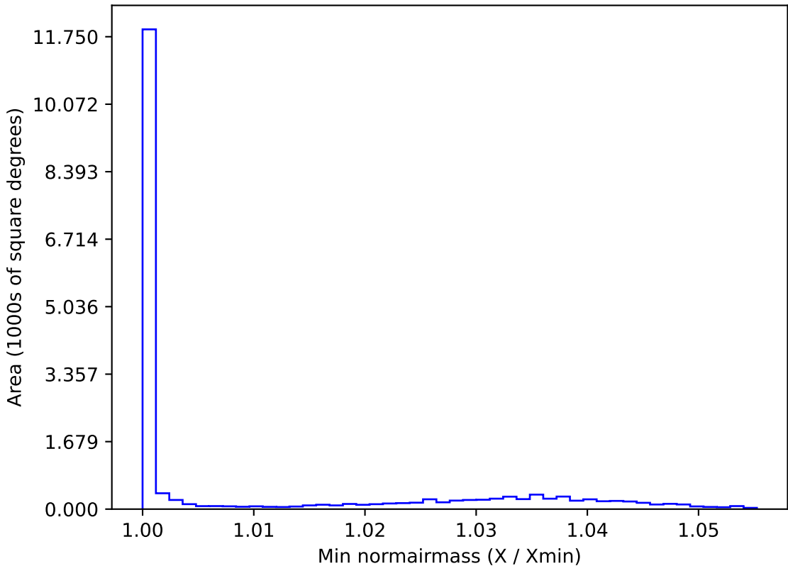
weather_cloudso14v3.4_10yrs WFD u band: Min normairmass
