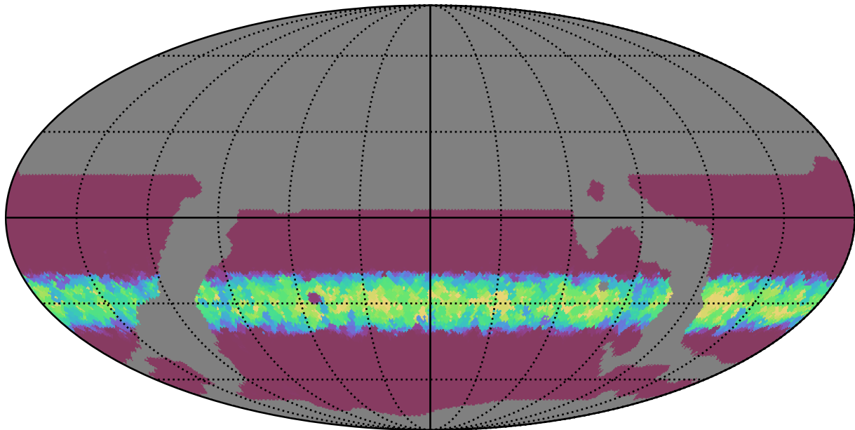
weather_cloudso14v3.4_10yrs WFD r band: Min normairmass
