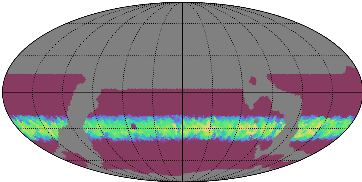
weather_cloudso14v3.4_10yrs WFD i band: Min normairmass
