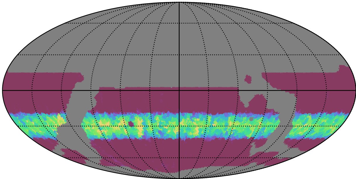
weather_cloudso14v3.4_10yrs WFD g band: Min normairmass
