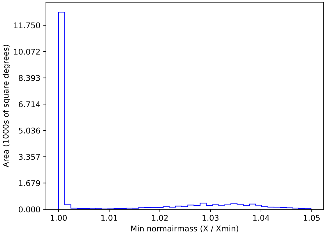
weather_cloudso14v3.4_10yrs WFD g band: Min normairmass
