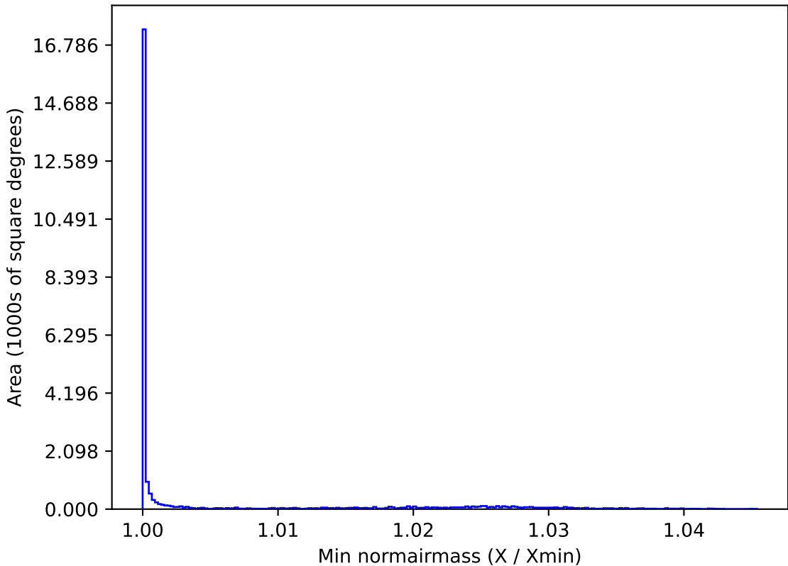
weather_cloudso14v3.4_10yrs All sky z band: Min normairmass
