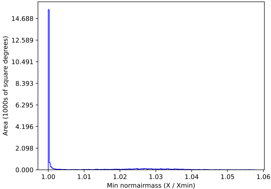
weather_cloudso14v3.4_10yrs All sky y band: Min normairmass
