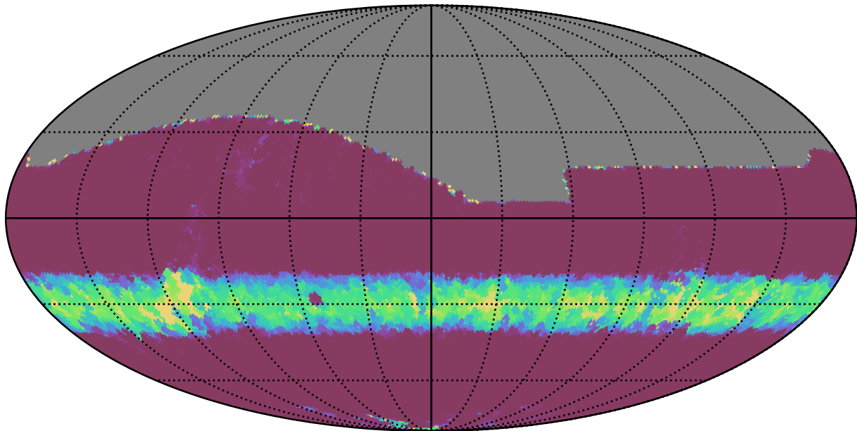
weather_cloudso14v3.4_10yrs All sky i band: Min normairmass
