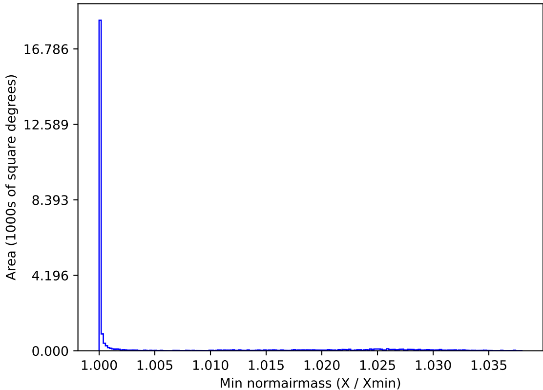
weather_cloudso14v3.4_10yrs All sky i band: Min normairmass
