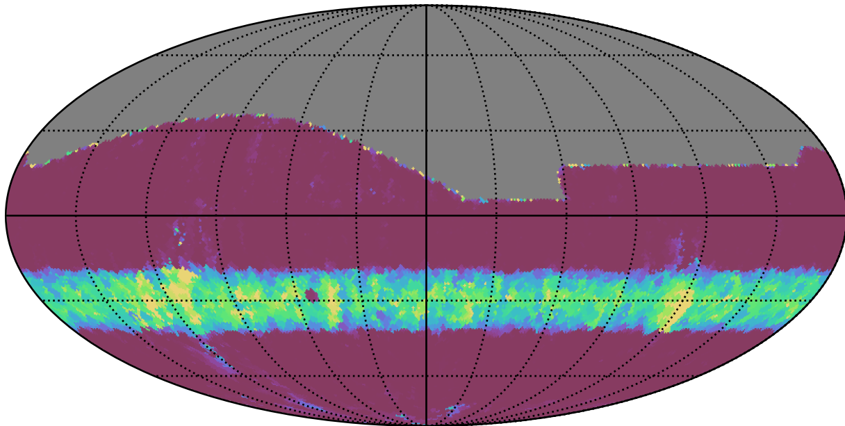
weather_cloudso14v3.4_10yrs All sky g band: Min normairmass
