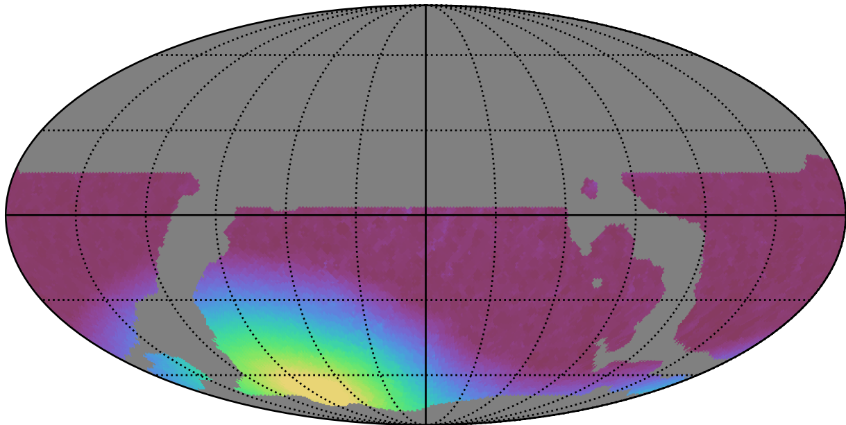
weather_cloudso14v3.4_10yrs WFD y band: Min moonDistance
