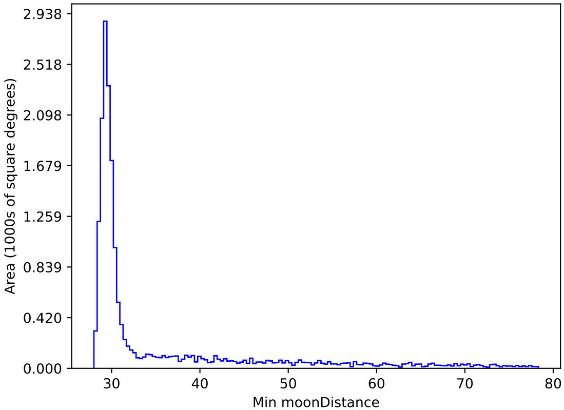
weather_cloudso14v3.4_10yrs WFD y band: Min moonDistance
