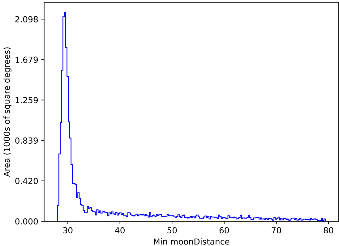
weather_cloudso14v3.4_10yrs All sky y band: Min moonDistance
