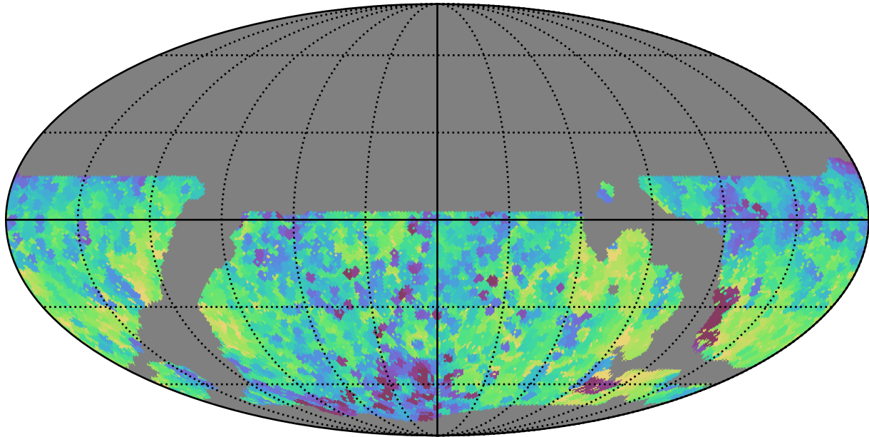
weather_cloudso14v3.4_10yrs WFD y band: Min fiveSigmaDepth
