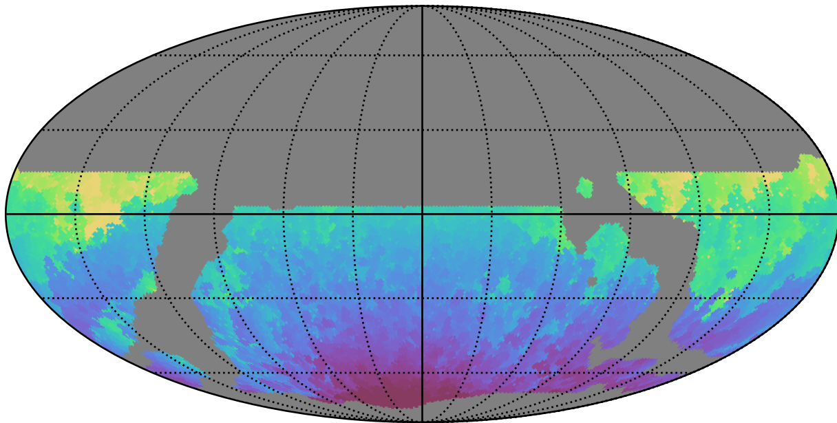
weather_cloudso14v3.4_10yrs WFD z band: Min HA
