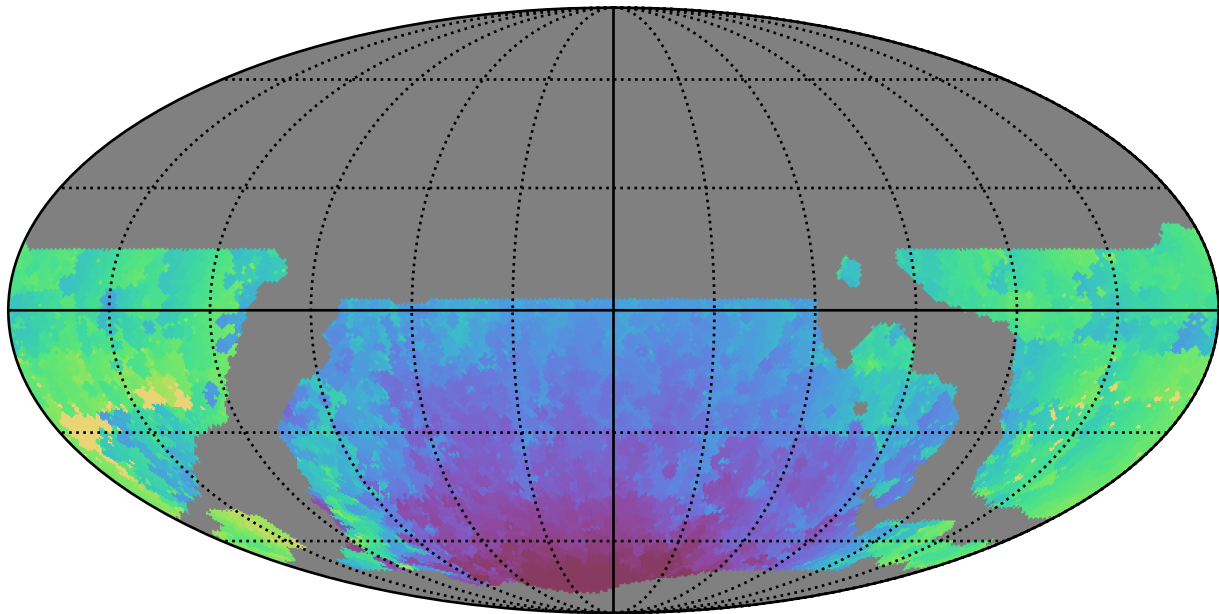
weather_cloudso14v3.4_10yrs WFD y band: Min HA
