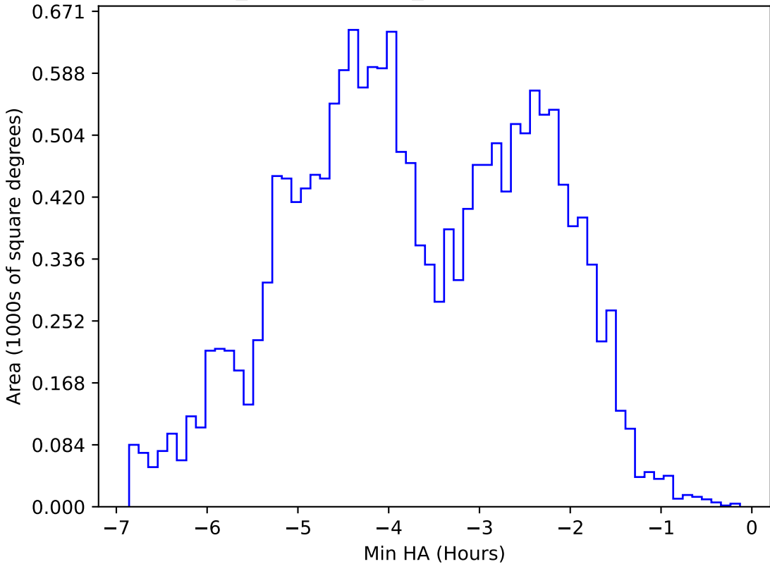
weather_cloudso14v3.4_10yrs WFD y band: Min HA
