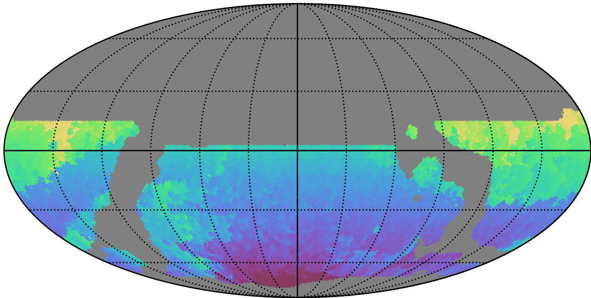
weather_cloudso14v3.4_10yrs WFD r band: Min HA
