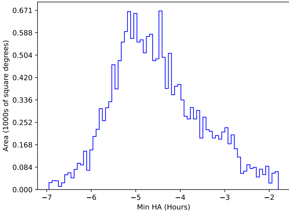
weather_cloudso14v3.4_10yrs WFD r band: Min HA
