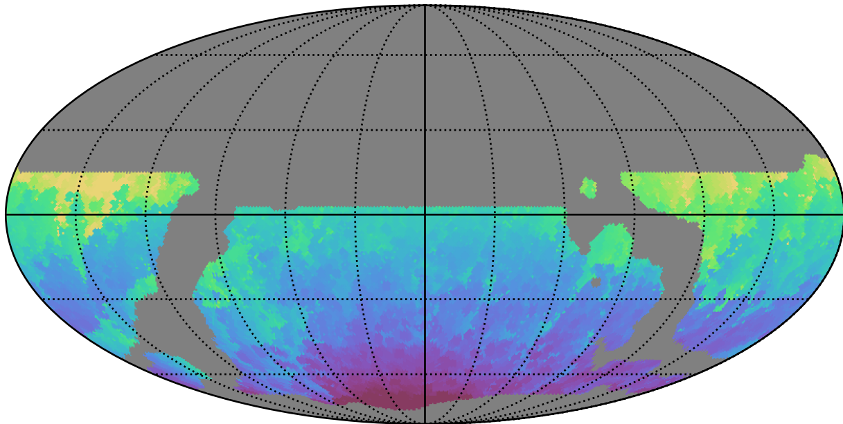
weather_cloudso14v3.4_10yrs WFD i band: Min HA
