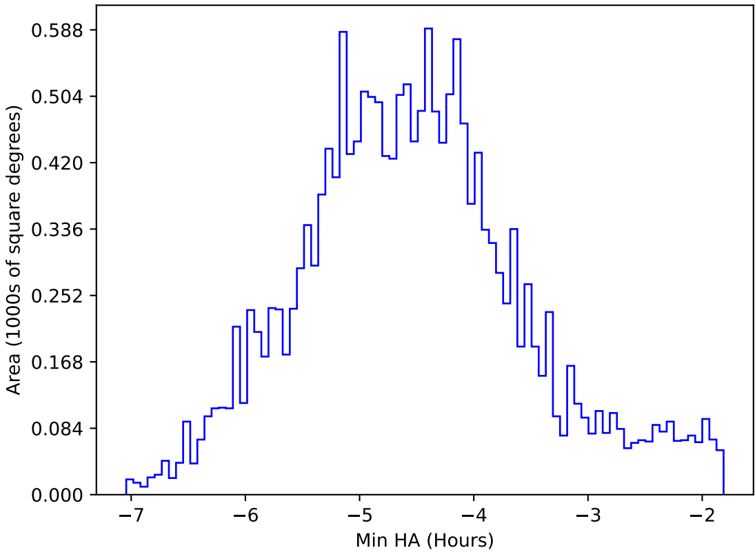
weather_cloudso14v3.4_10yrs WFD i band: Min HA
