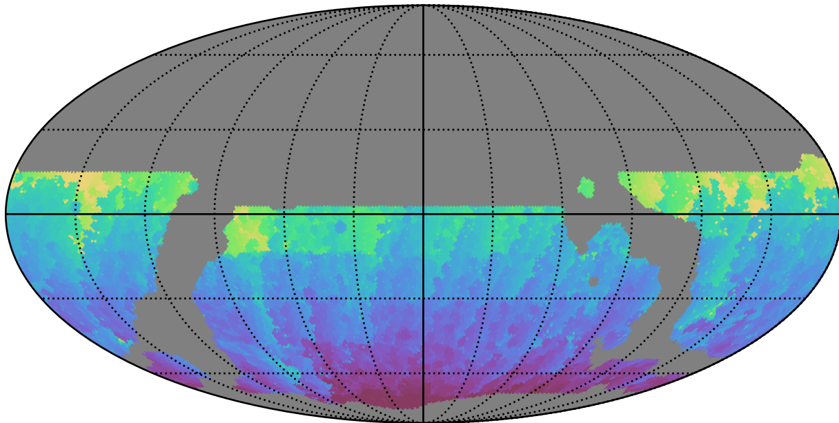
weather_cloudso14v3.4_10yrs WFD g band: Min HA
