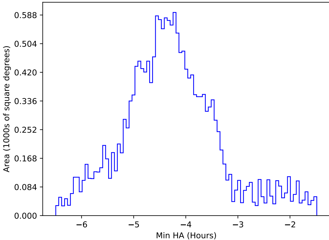
weather_cloudso14v3.4_10yrs WFD g band: Min HA
