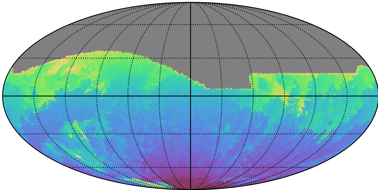
weather_cloudso14v3.4_10yrs All sky z band: Min HA
