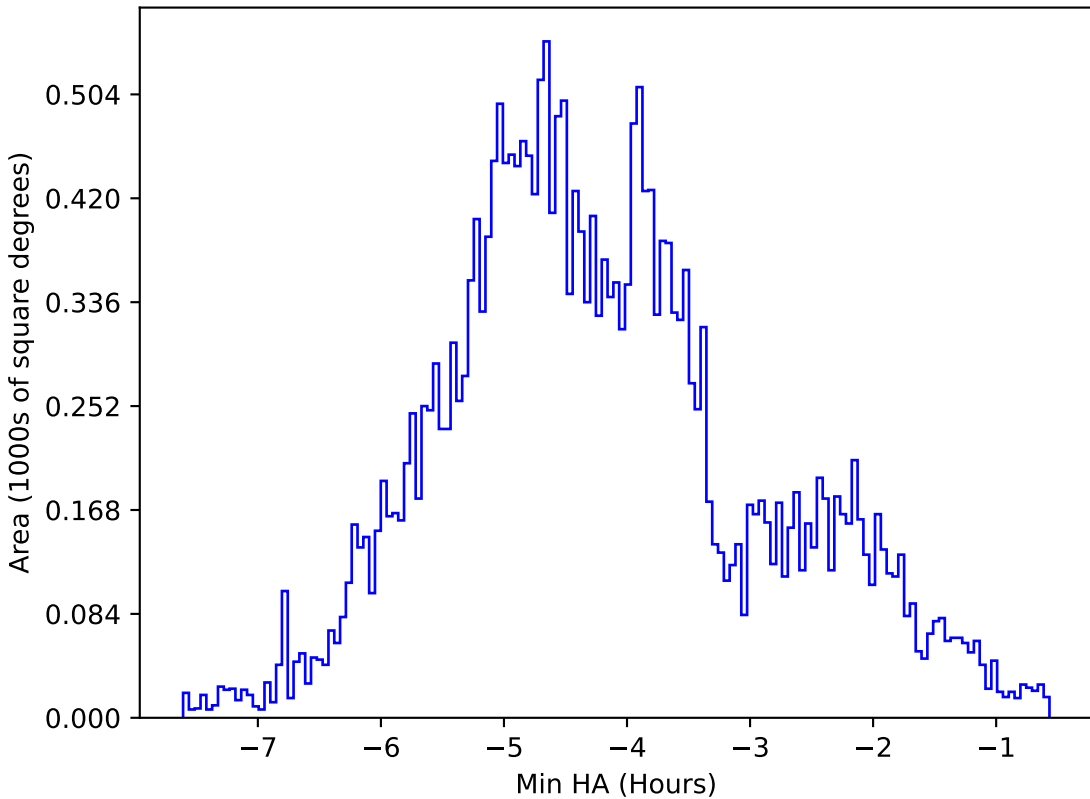
weather_cloudso14v3.4_10yrs All sky z band: Min HA
