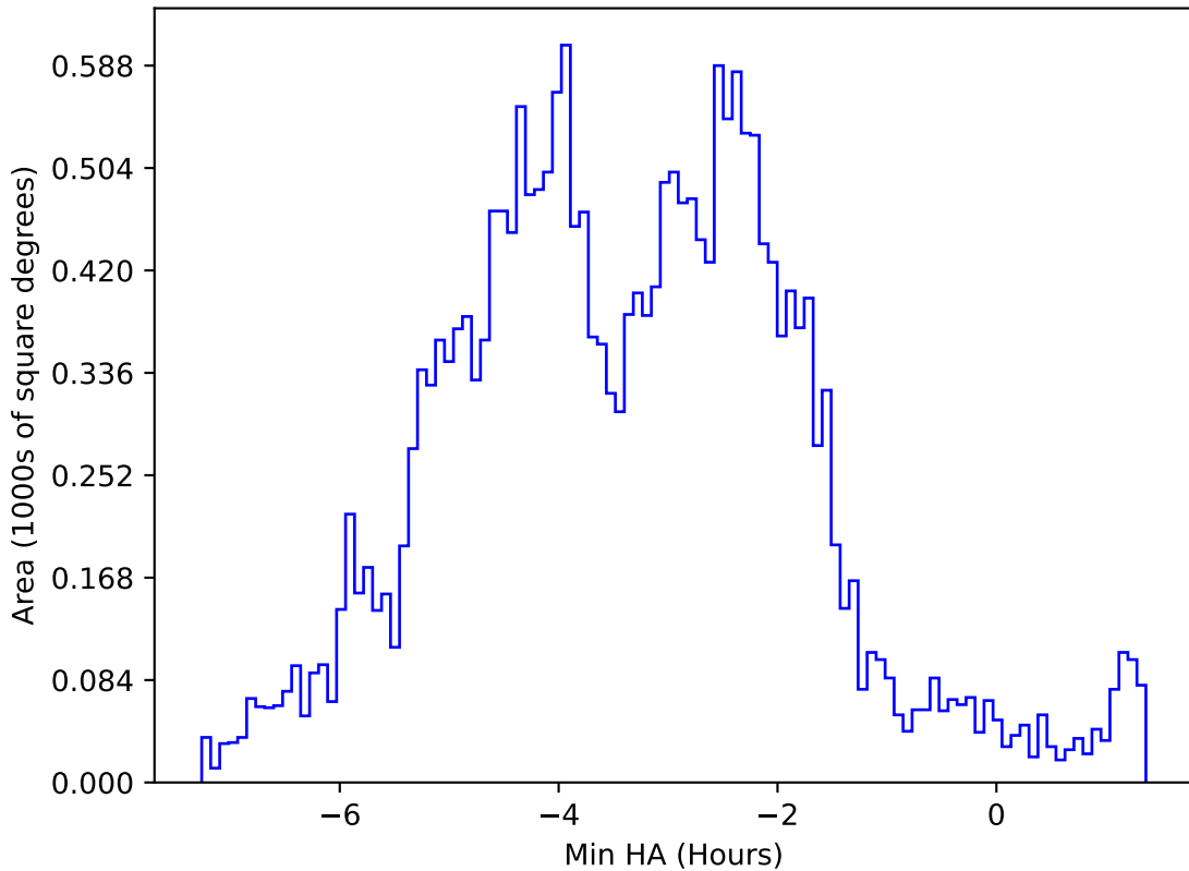
weather_cloudso14v3.4_10yrs All sky y band: Min HA
