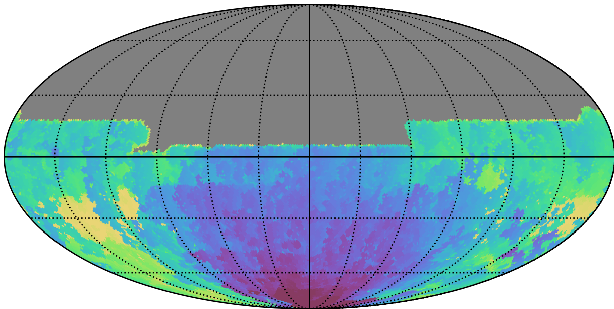
weather_cloudso14v3.4_10yrs All sky u band: Min HA
