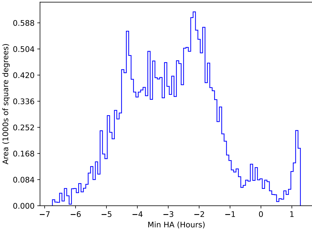
weather_cloudso14v3.4_10yrs All sky u band: Min HA
