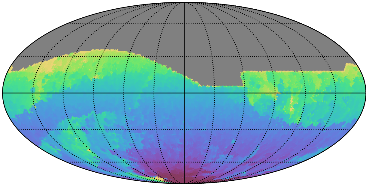
weather_cloudso14v3.4_10yrs All sky r band: Min HA
