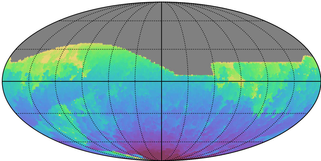
weather_cloudso14v3.4_10yrs All sky i band: Min HA
