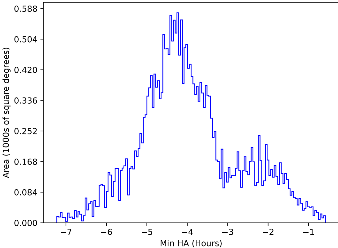
weather_cloudso14v3.4_10yrs All sky g band: Min HA
