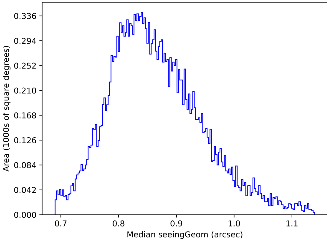
weather_cloudso14v3.4_10yrs Yr 1 y band: Median seeingGeom
