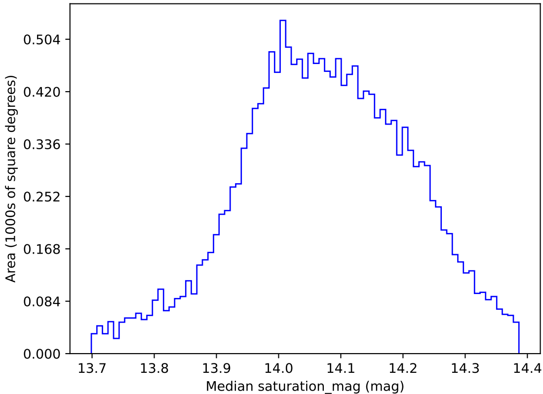
weather_cloudso14v3.4_10yrs WFD z band: Median saturation_mag
